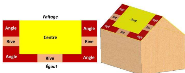
TOITURE A DEUX VERSANTS
