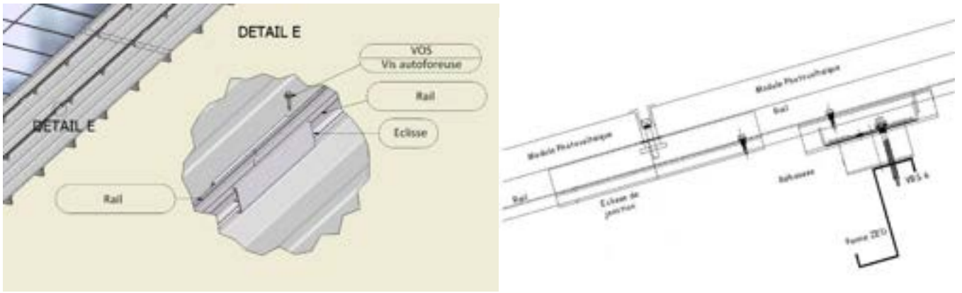
Figure 24 – Éclissage à la jonction de deux rails
