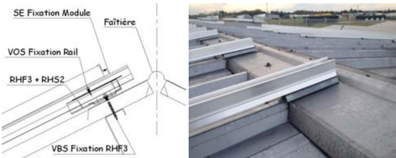
Positionnement des rehausse de faîtière : une seule par colonne de rails
