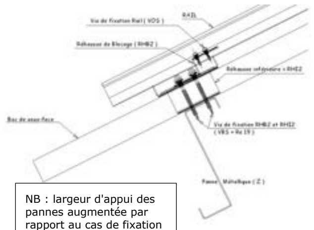
Cas de fixation avec 2 vis VBS et 2 vis VOS
