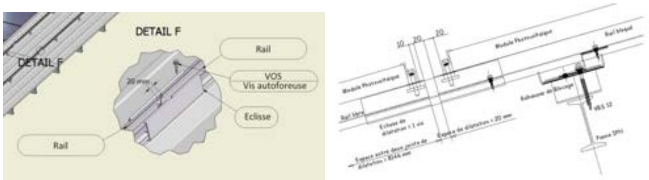
Figure 25 – Éclissage au joint de dilatation
