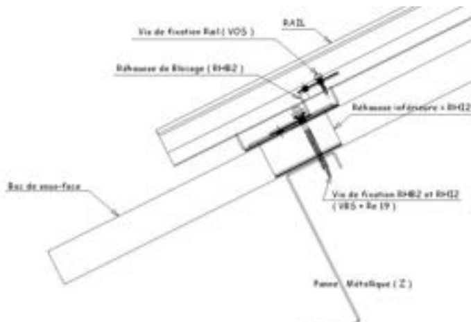
Cas de fixation avec 1 vis VBS et 1 vis VOS
