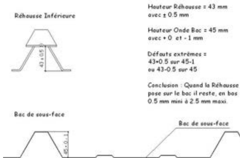
Figure 13 – Illustration des tolérances dimensionnelles entre rehausse / nervure de bac / cale intercalaire d'onde
