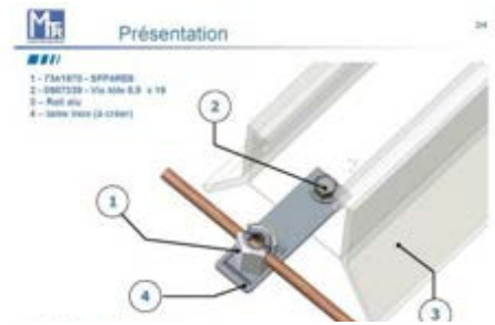
Bornier déporté SOLFIL
