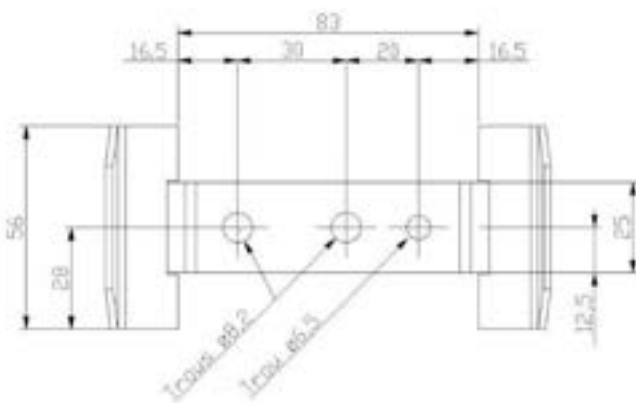
Figure 7 – Rehausse de faitage
