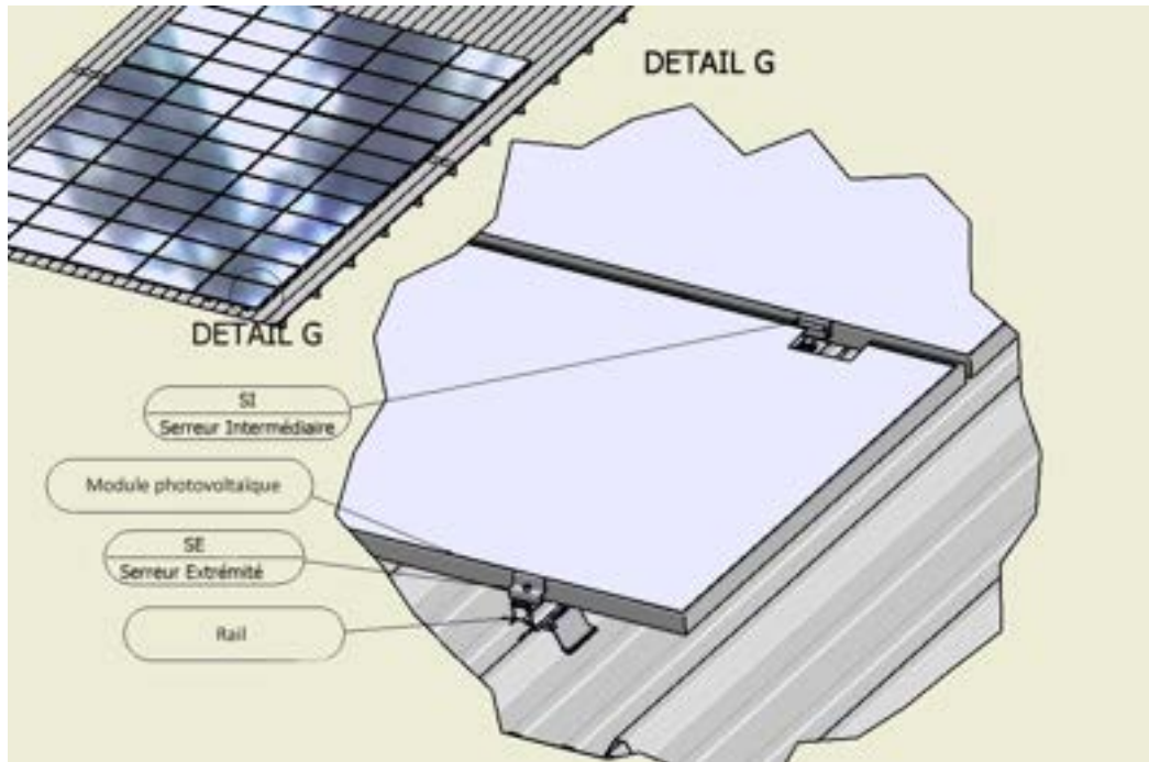
Figure 26 – Mise en place des modules avec les serreurs intermédiaires (SI) ou d'extrémité (SE)
