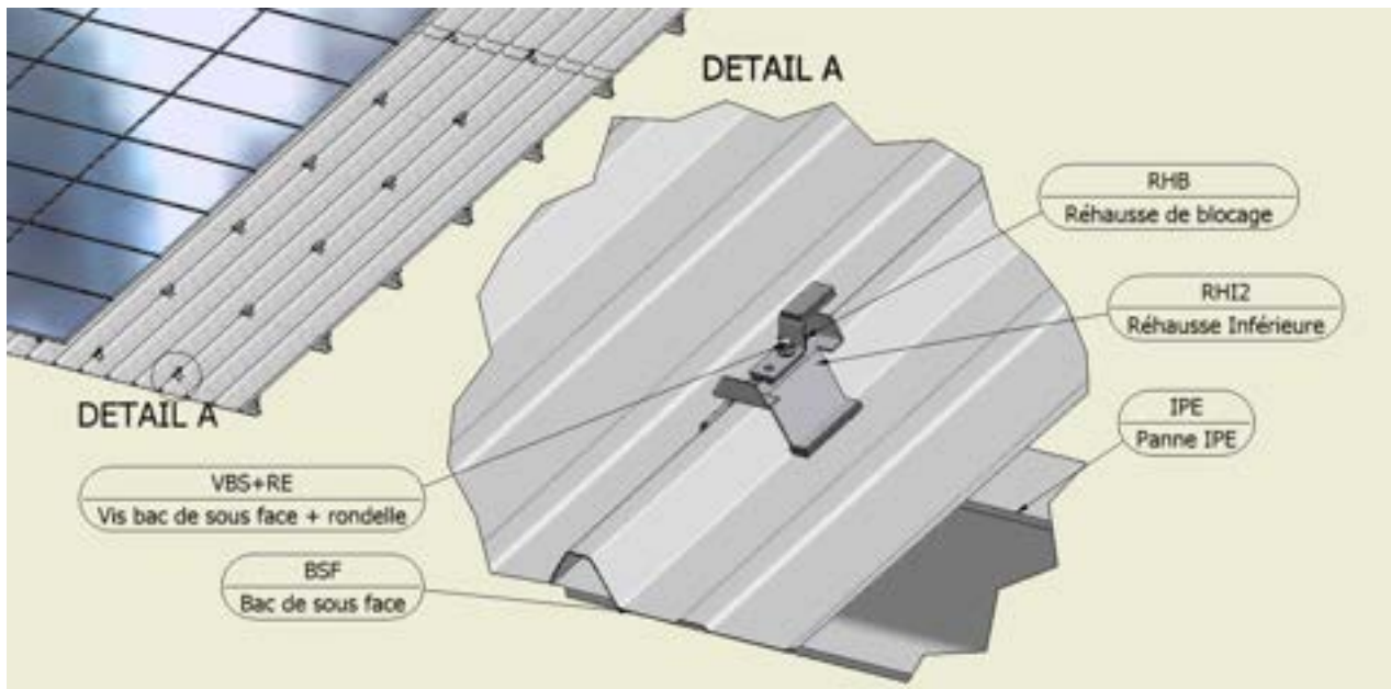
Figure 18 - Illustration de la fixation des bacs de sous-face à l'aide des rehausse inférieures avec la rehausse de blocage
