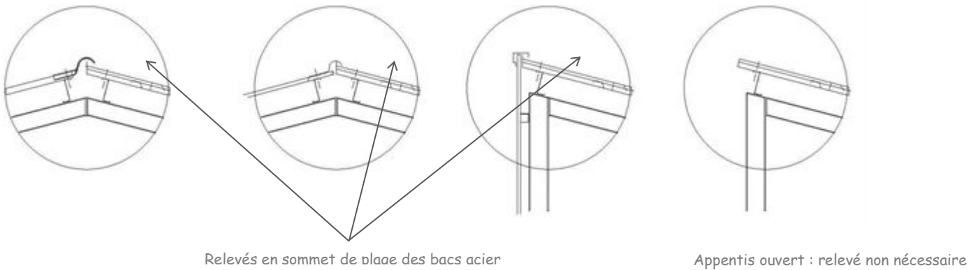
Cas avec Bavette d'étanchéité supérieure « Fibrociment » ou « sous coiffe »
