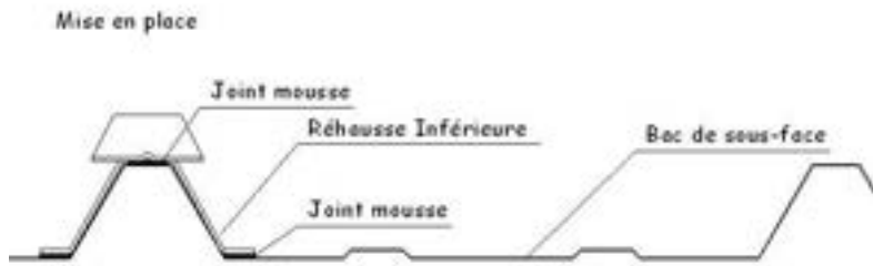
Figure 17 – Mise en place de la rehausse inférieure
