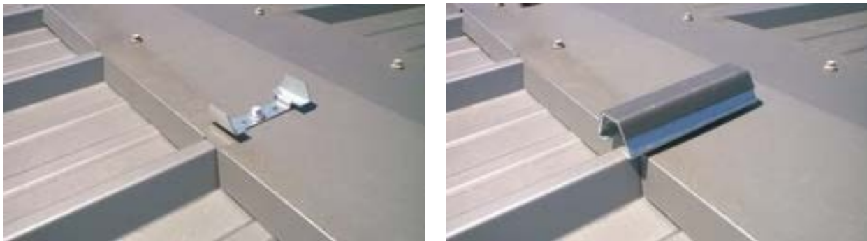
Figure 19 - Illustration de l'utilisation de la rehausse de faîtière
