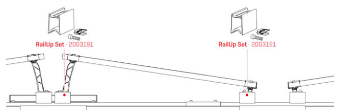
Version D-DOME 6 CLASSIC avec RailUp
