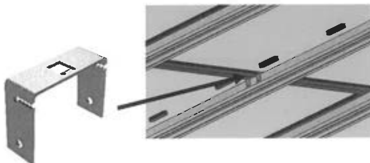
Vues de l'assemblage crapaud retour cadre/ module pour rail intermédiaire
