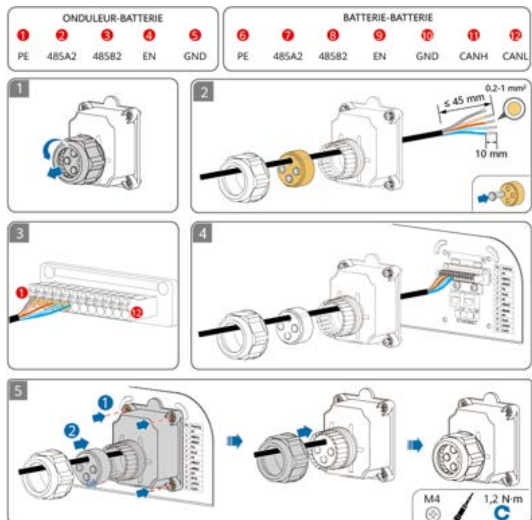
Figure 5-6 Connexions du port de signal
