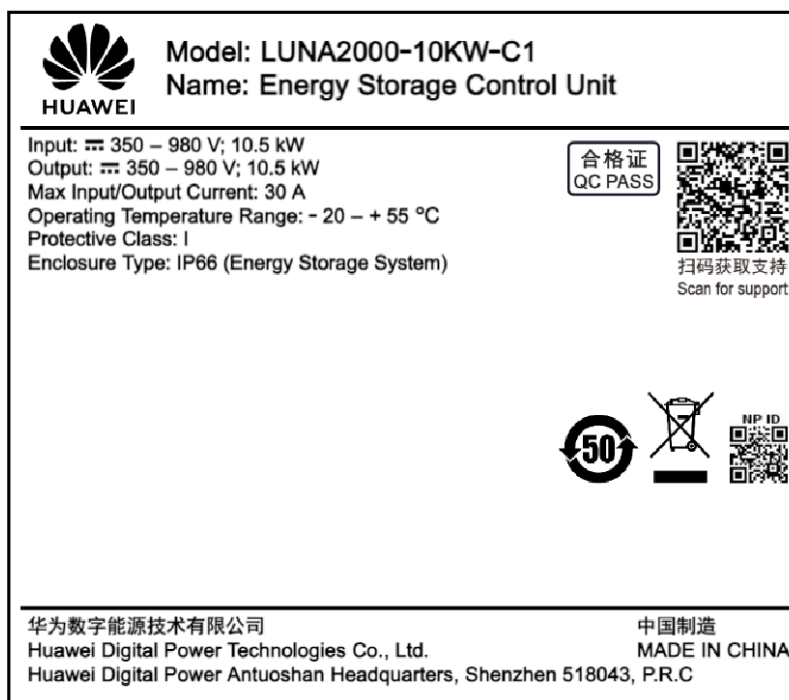
Figure 2-11 Plaque signalétique d'une unité de contrôle du stockage de l'énergie
