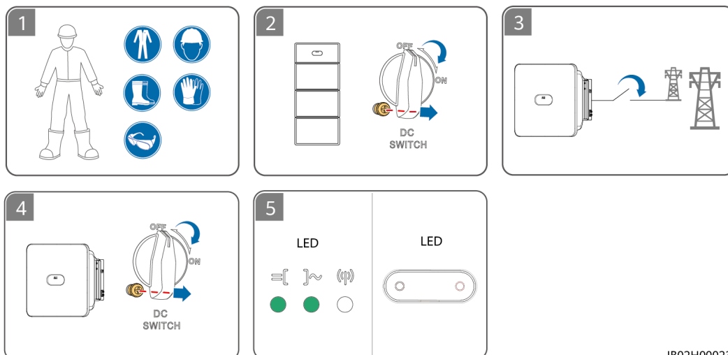
Figure 6-1 Processus d'allumage
