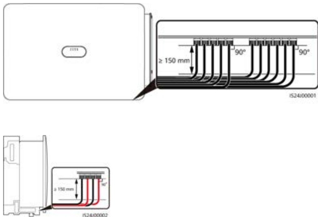
Figure 5-14 Exigences en matière de câblage d'alimentation d'entrée CC
