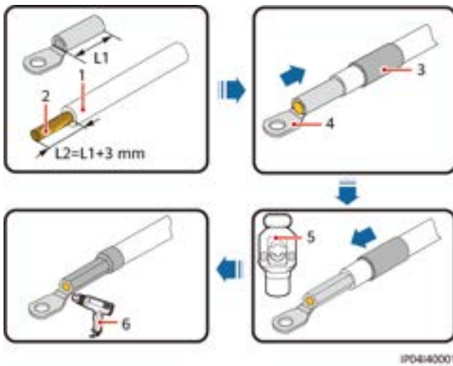
Figure D-3 Sertissage d'une borne DT
