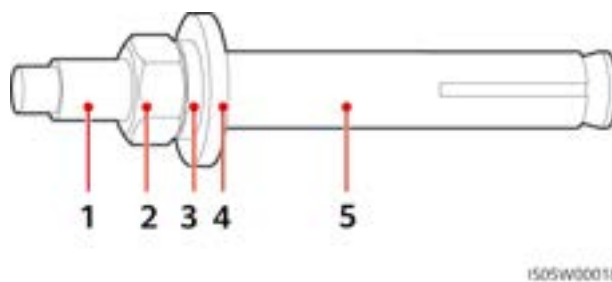
Figure 4-14 Structure d'un boulon à expansion
