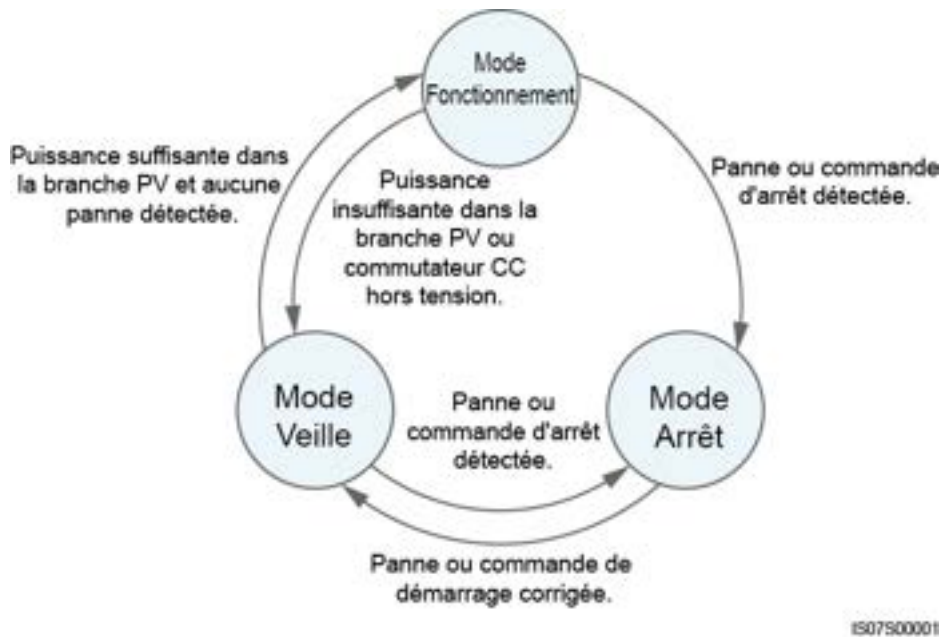
Figure 2-10 Modes de fonctionnement
