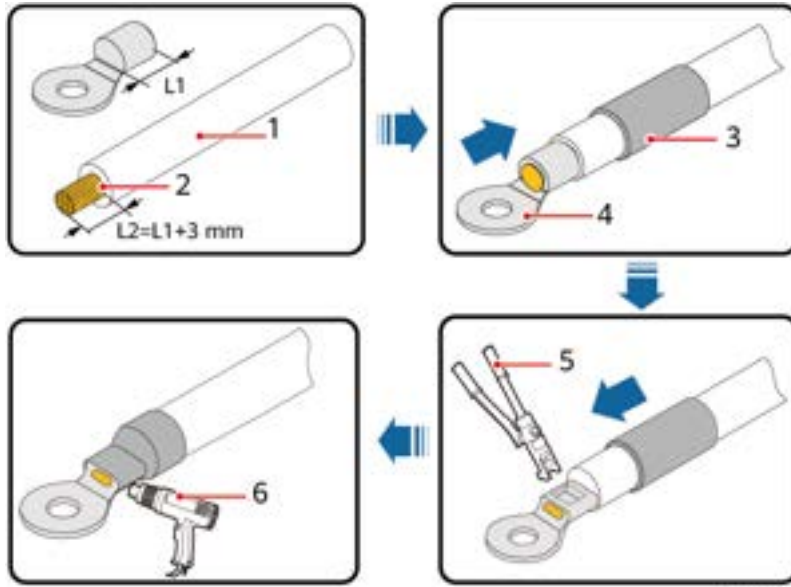
Figure D-2 Sertissage d'une borne OT
