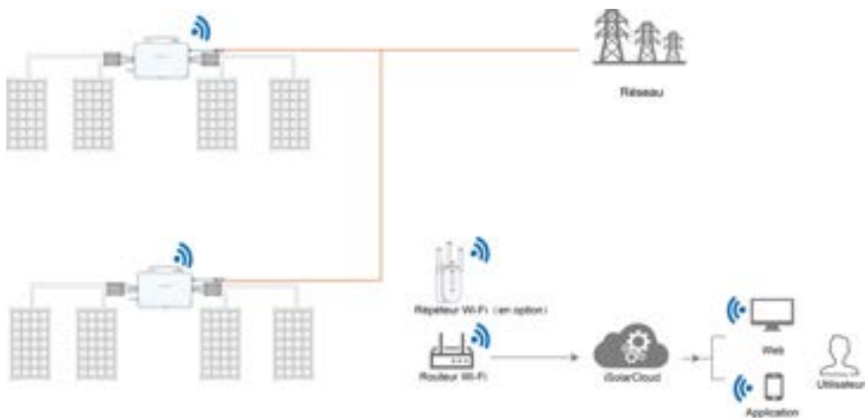
Figure 2-3 Schéma de raccordement au réseau d'un système PV monté sur toiture
