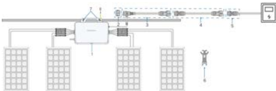
Figure 4-1 Accessoires pour système PV monté sur toiture
