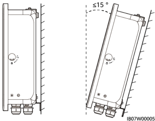
Figure 4-3 Angle d'installation
