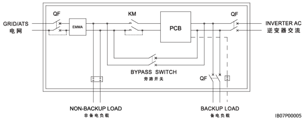
Figure 2-9 Schéma électrique du SmartGuard
