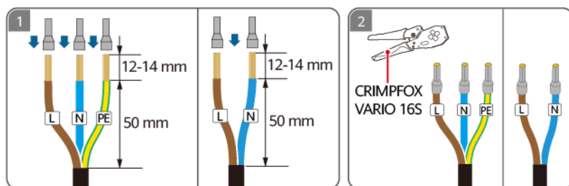
Figure 5-6 Sertissage des bornes d'extrémité du cordon CA
