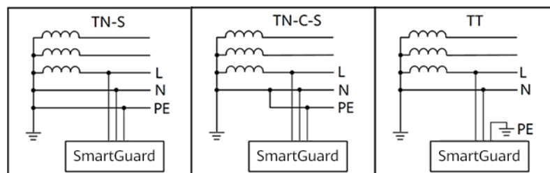
Figure 2-6 Systemes de mise à la terre
