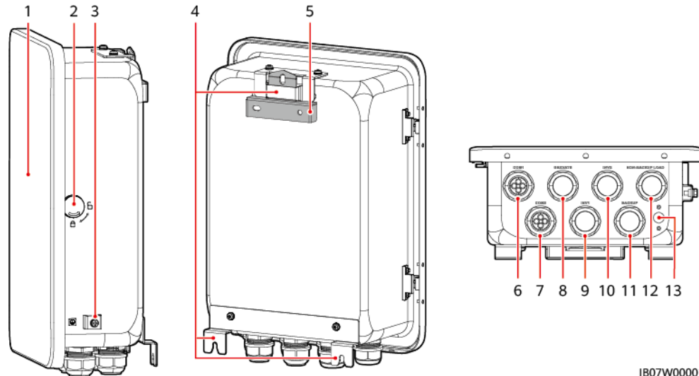
Figure 2-7 Aspect visuel et ports
