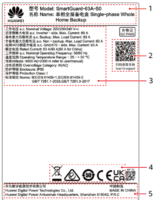
Figure 2-11 Plaque signalétique (SmartGuard-63A-S0 par exemple)
