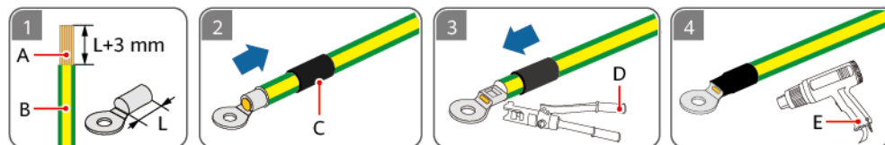
Figure 5-2 Sertissage d'une borne OT
