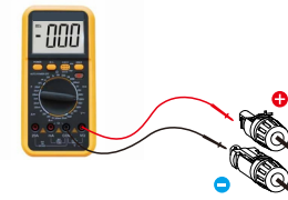
Figure 5.16 Mesure du multimètre
