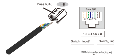
Figure 5.30 Dénudez la couche isolante et connectez le câble à la prise RJ45
