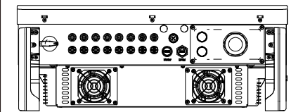
Figure 5.17 Connectez les connecteurs CC à l'onduleur
